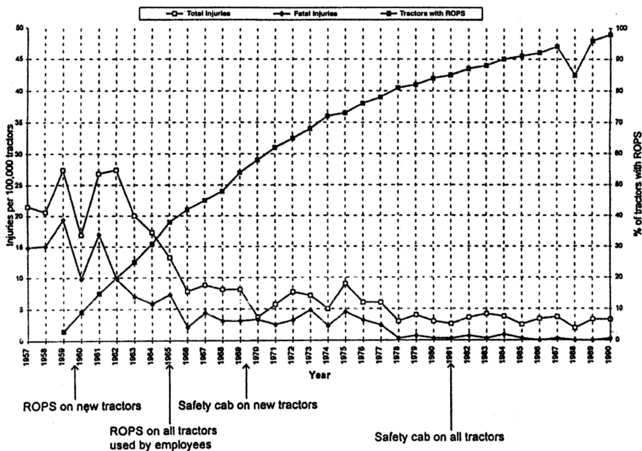
Figura 15. Infortuni da roll-over per 100.000 trattori in Svezia, 1957-1990*.
